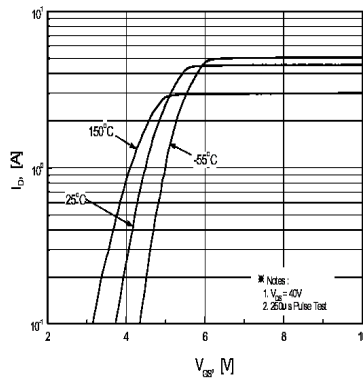
I_D - V_{GS}
